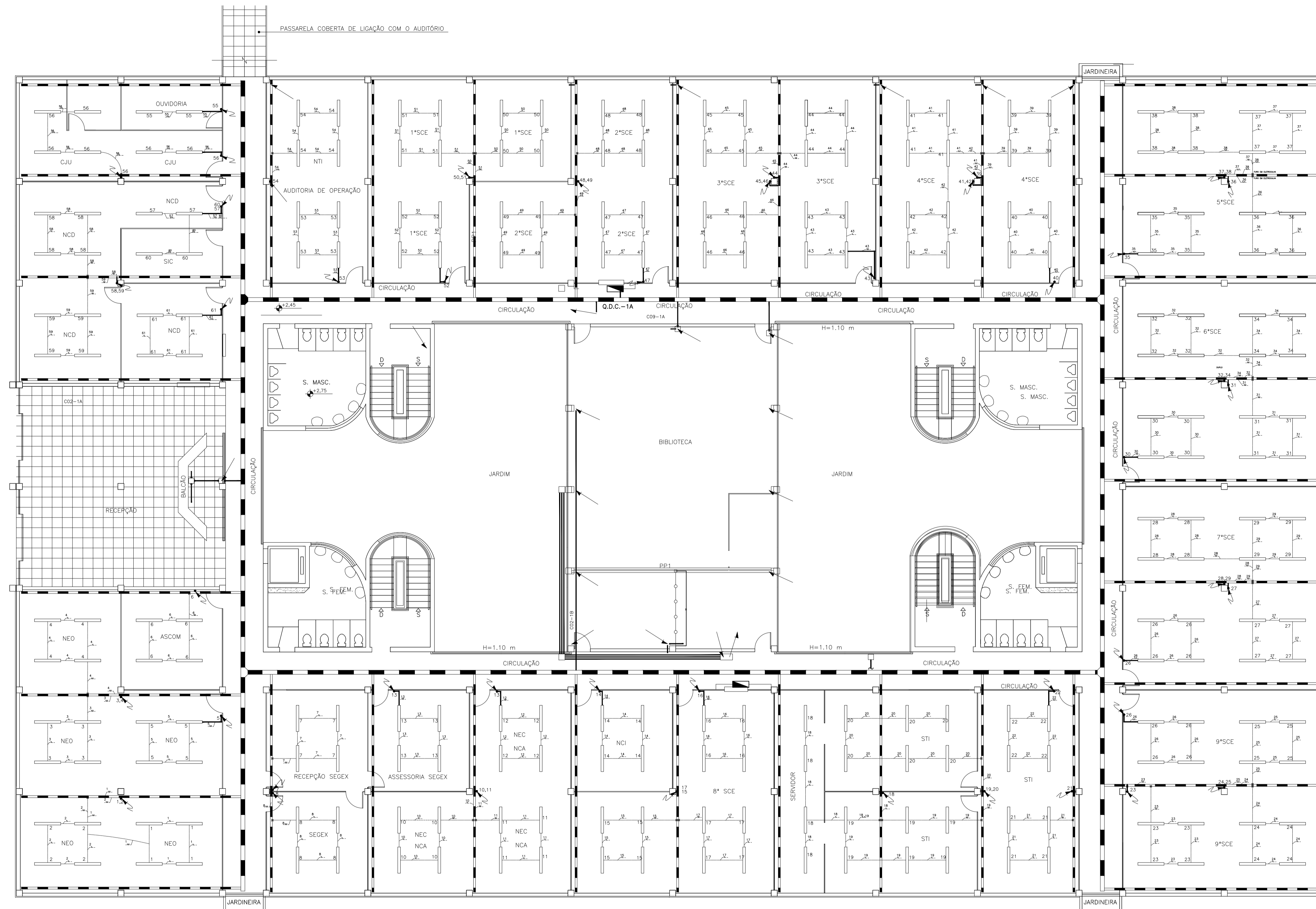
PLANTA BAIXA - 1º PAVIMENTO ESCALA: 1:100
